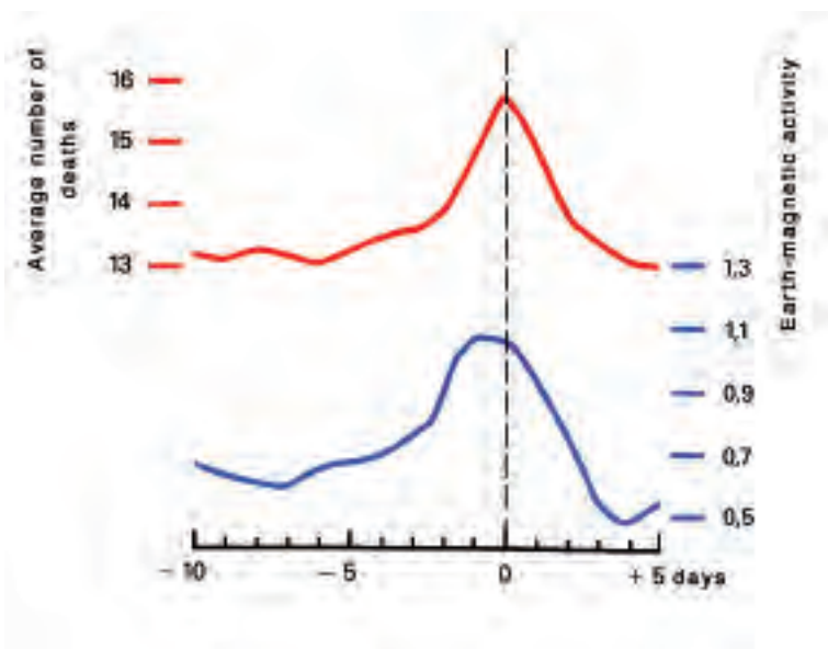
Illustration 8 : Tempêtes magnétiques (en bas) et mortalité due à des affections nerveuses et cardiovasculaires.
